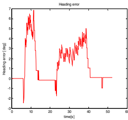
Fig. 15. Heading error, \theta_e
