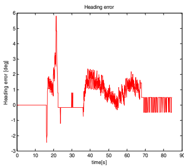
Fig. 9. Heading error, \theta_e
