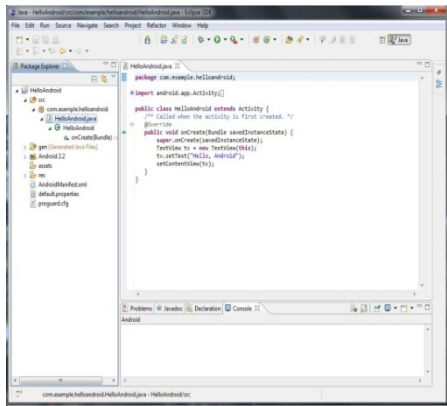
Fig. 4. Eclipse IDE
